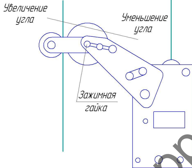
Рис.5. Схема настройки угла блокировки.
