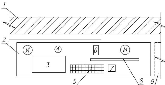
1 - утепляемая стена; 2 - люлька; 3 - плиты утеплителя; 4 - емкость с клеевым составом; 5 - рупон стеклосетки; 6 - ящик с инструментом; 7 - контейнер с дюбелями; 8 - уровень строительный; 9 - место перестановки люльки; И - рабочие места изолировщиков
