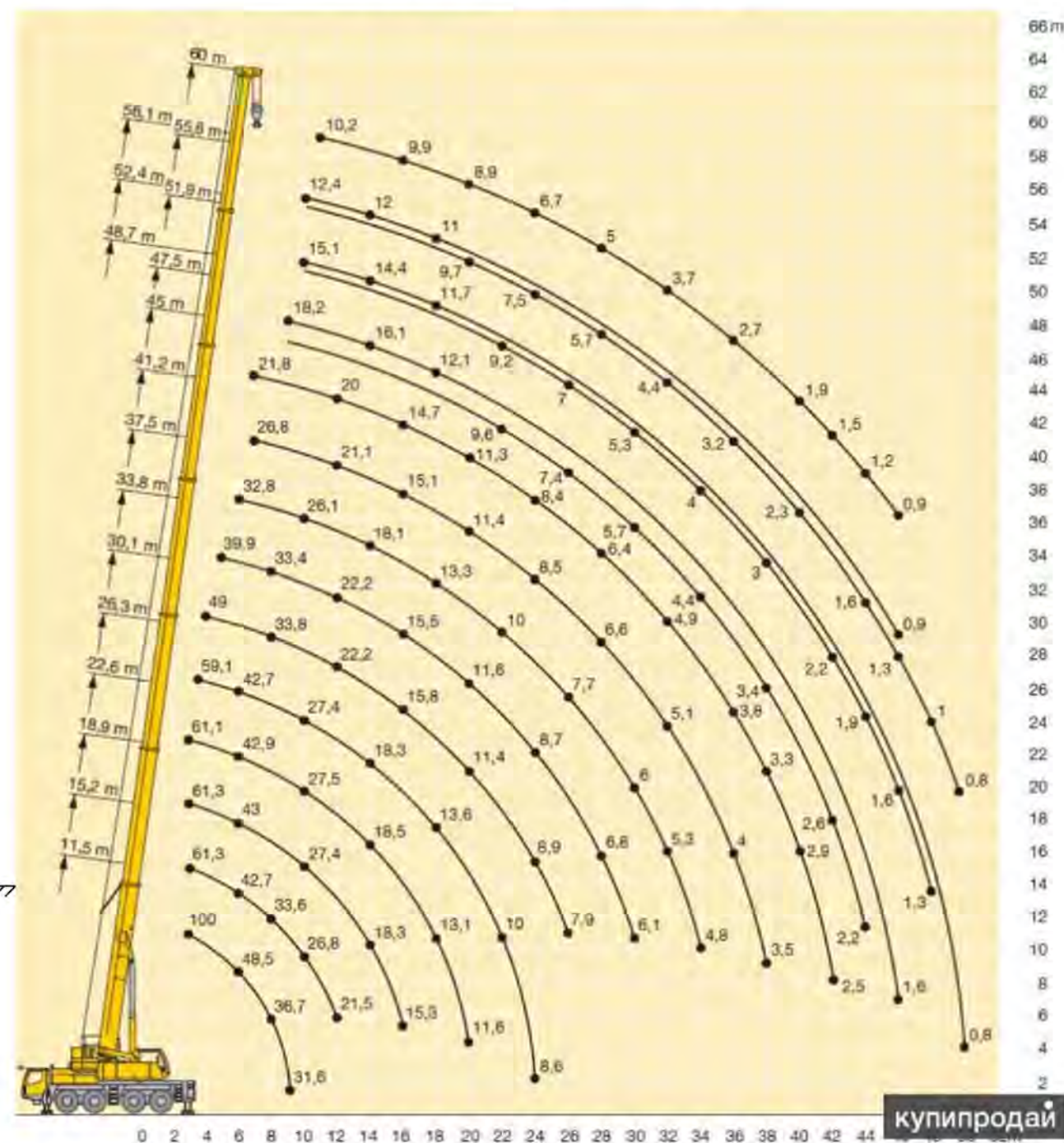
Технические характеристики LIEBHERR LTM 1100-4.2
