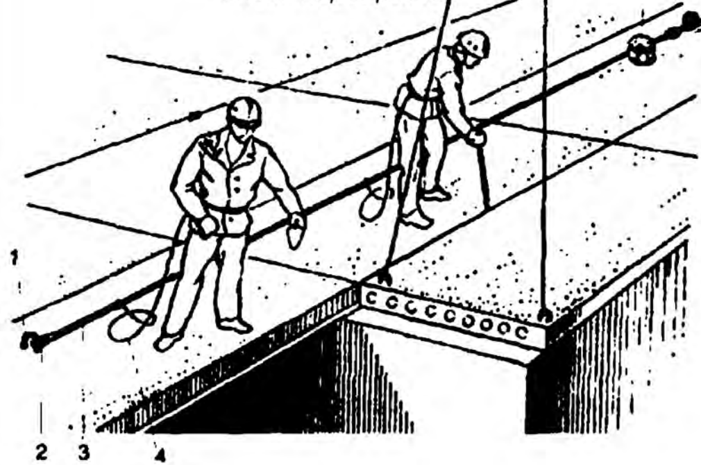
Схема страховки при монтаже плит перекрытия
