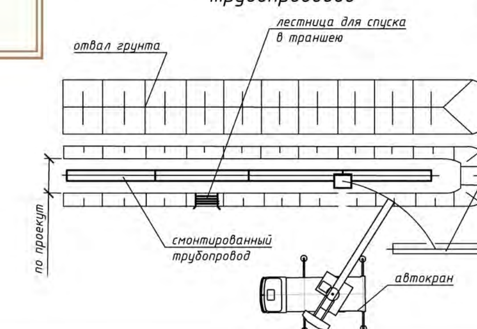
Схема производства работ по монтажу трубопроводов
