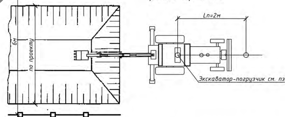
Схема забоя экскаватора-погрузчика при рытье траншеи
