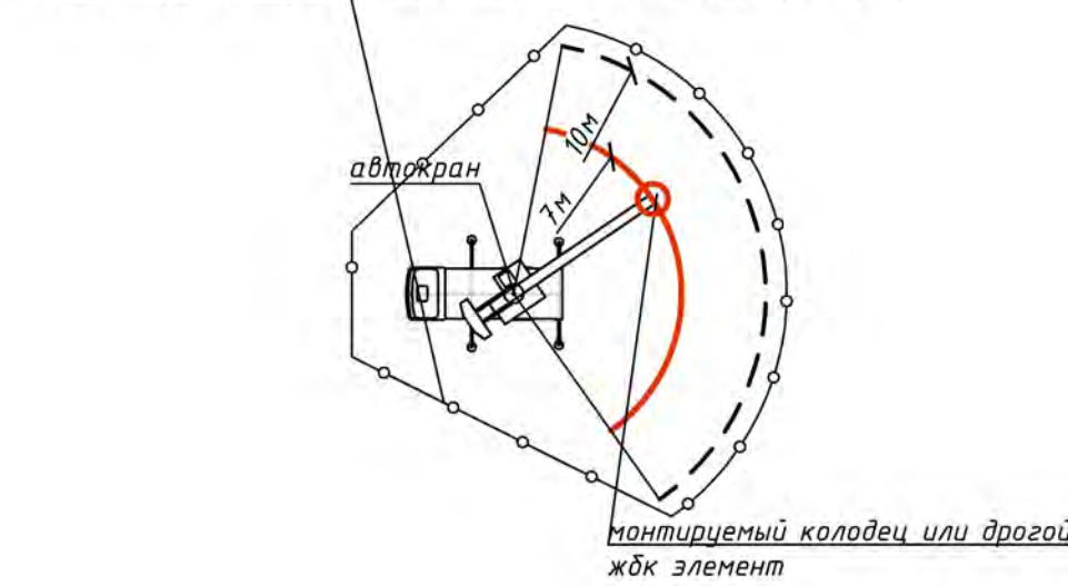
Выемка грунта погрузчиком
