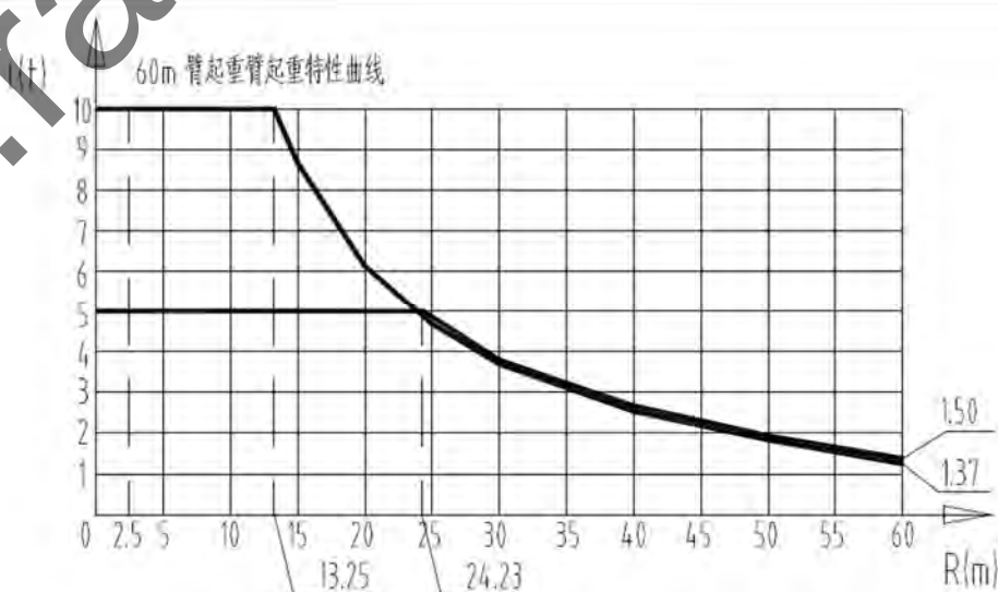
Технические характеристики Zoomlion TC6015A-10
