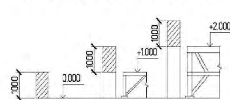
Схема производства погрузочно-разгрузочных работ вручную
