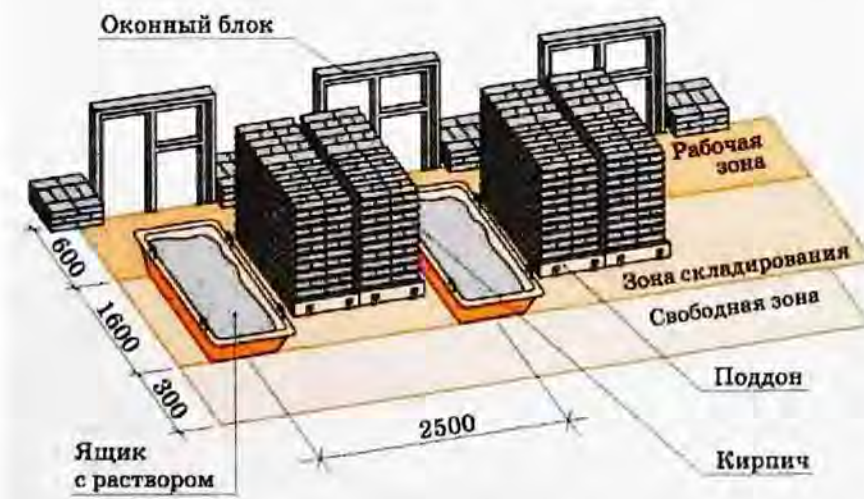
Схема производства работ с шарнирно-панельных подмостей
