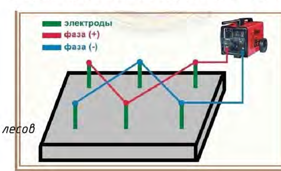
Схема электропрогрева бетона вертикальными электродами
