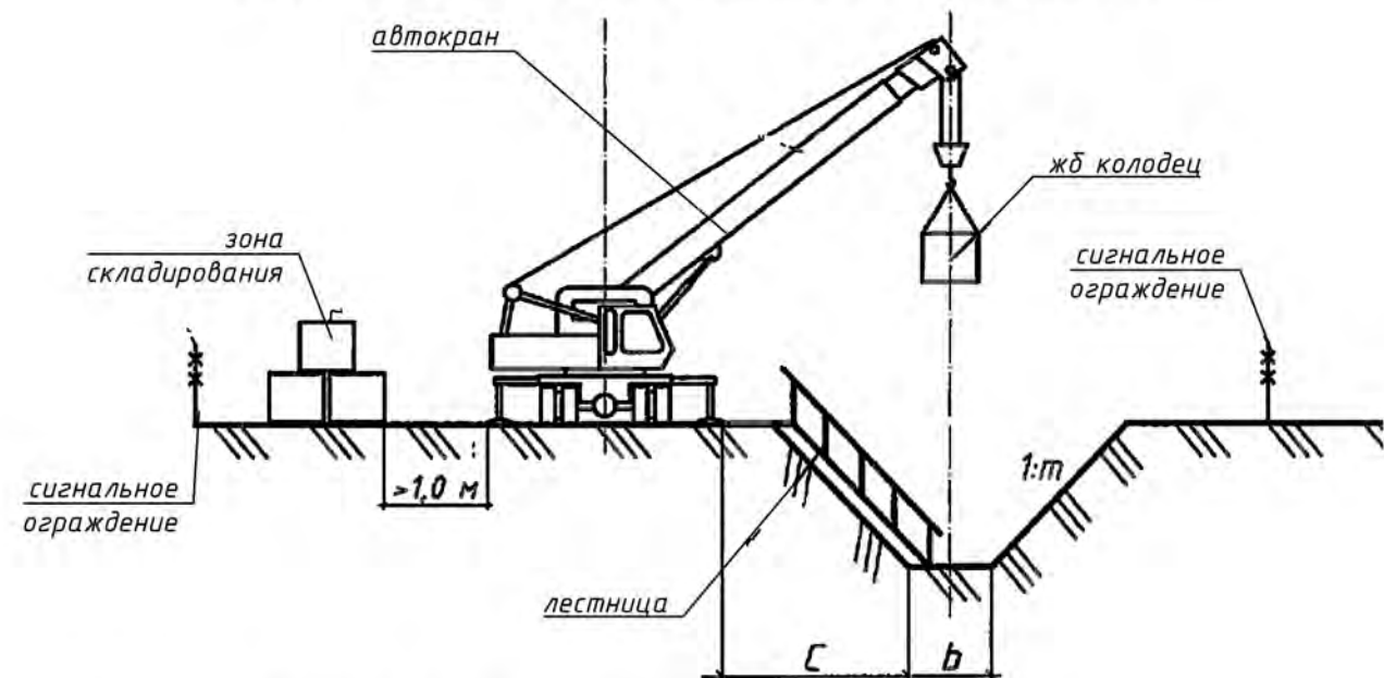
Схема монтажа жб колодцев автокраном
