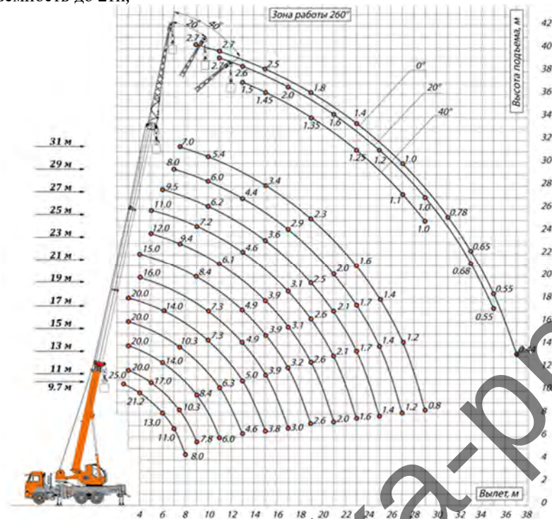
Характеристики автокрана
